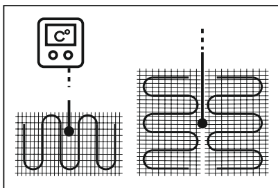
Рис. 5 – Установка датчика температуры пола между витками кабеля
