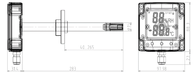
Размеры датчика, мм
