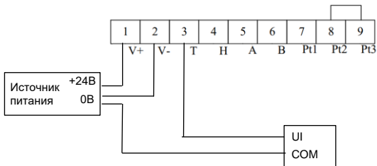
Схема подключения выхода температуры 0...10 В пост. тока
