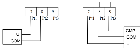
Выход NTC 10K 2-проводная схема
