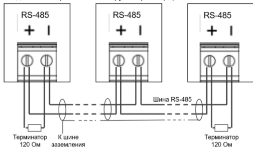
Подключение шины RS-485
