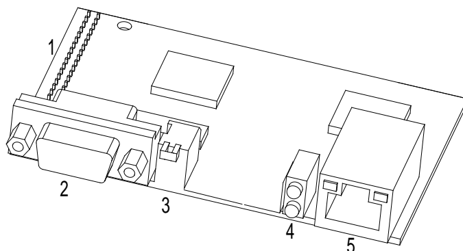
Рис. C.2 Внешний вид адаптера TX
