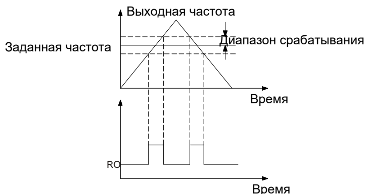
Рис. 5.24 Диаграмма диапазона достижения заданной частоты
