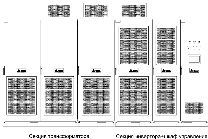
Рис. 2.6 Габаритные размеры
