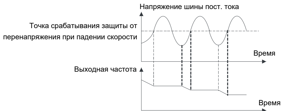
Рис. 5.34 Схема защиты от перегрузки по напряжению при потере скорости
