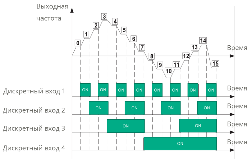
Рис. 5.29 Действие режима многоступенчатого регулирования скорости
