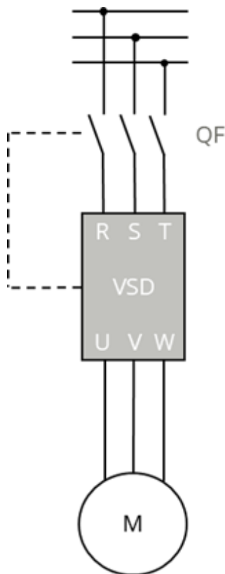
Рис. 4.1 Схема силовой цепи
