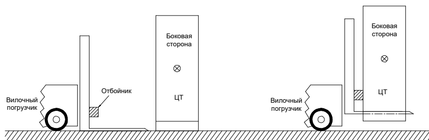
Рис. 8.3: Перемещение при помощи вилочного погрузчика
