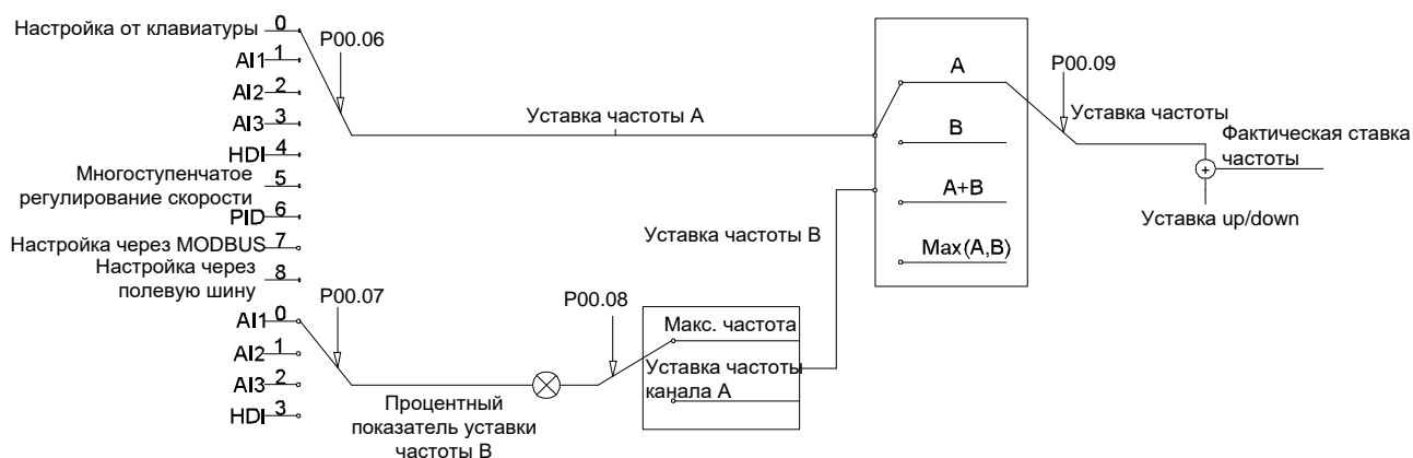
Рис. 5.1 Комбинация источников задания частоты
