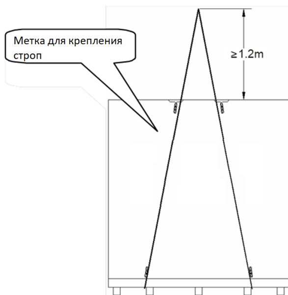
Рис. 8.1 Подъем оборудования в упаковке
