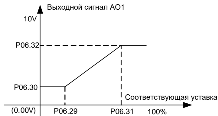
Рис. 5.21 Соотношение между аналоговым выходным сигналом и соответствующей уставкой
