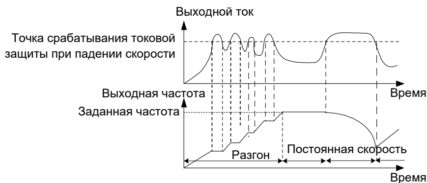
Рис. 5.35 Уровень автоматического ограничения тока
