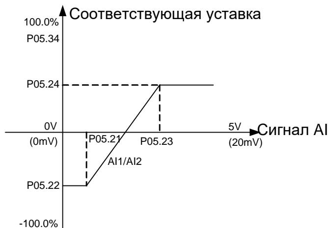
Рис. 5.19 Соотношение между сигналами AI1/AI2 и соответствующими уставками
