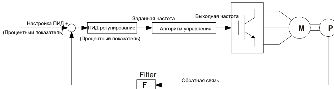
Рис. 5.26 Блок-схема ПИД-регулятора
