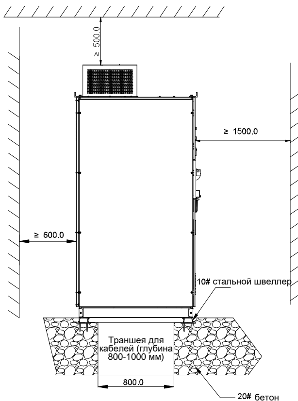
Рис. 8.6 Монтажная схема 2 (вид сбоку, ед. измерения: мм)
