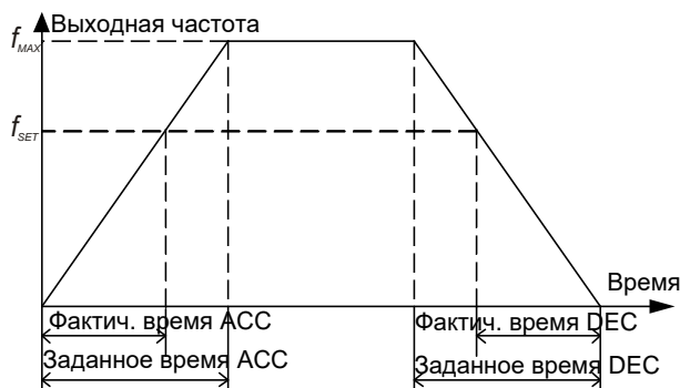
Рис. 5.2 Длительность ускорения и торможения
