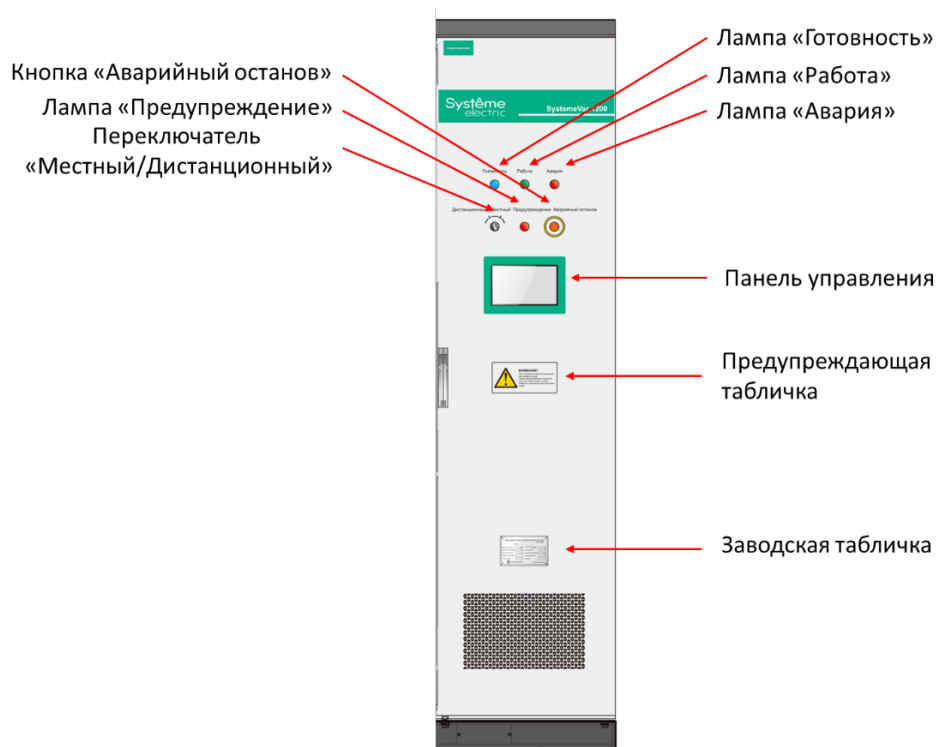
Рис. 3.12 Схема расположения панели оператора на двери шкафа управления
