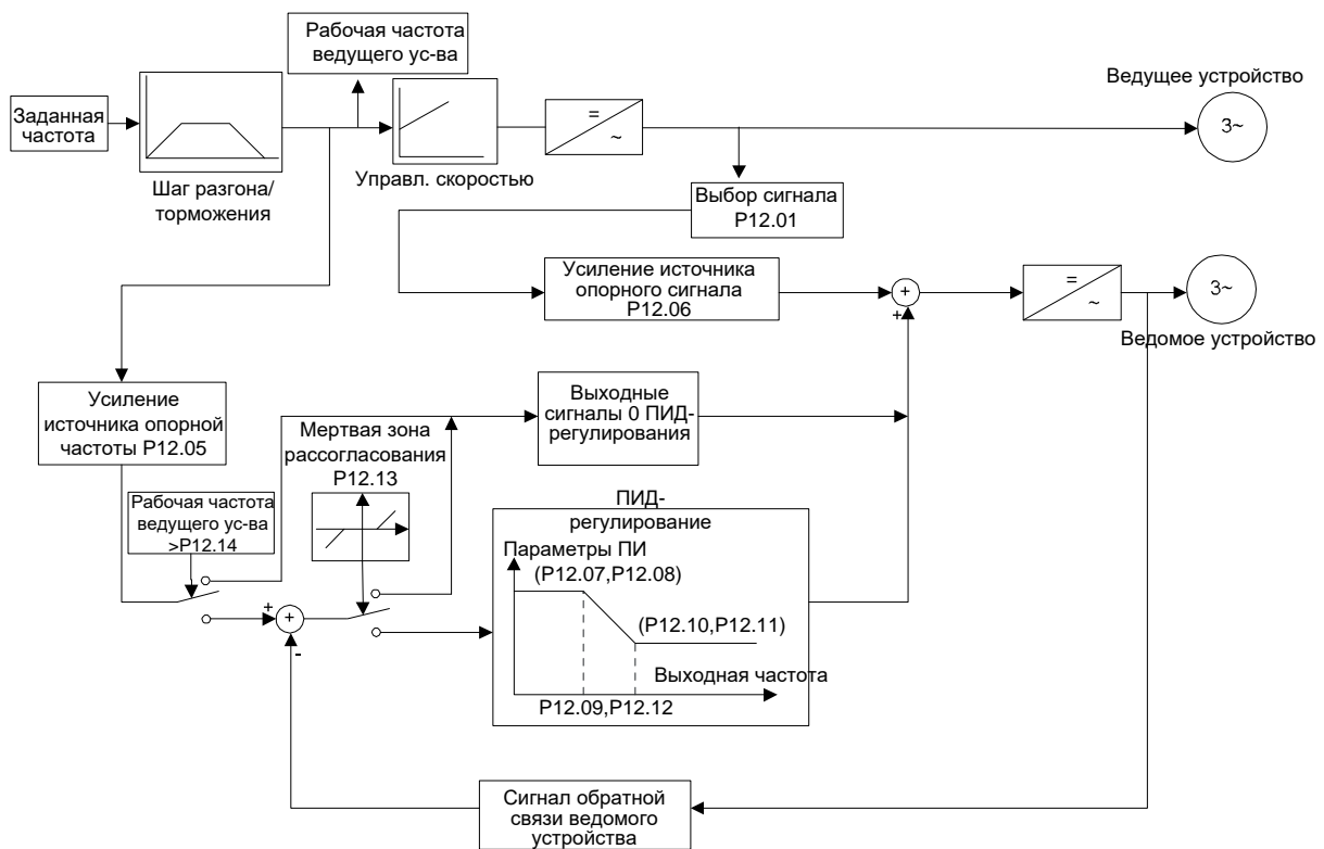
Рис. 5.31 Схема жесткого подключения «ведущее-ведомое устройство», ведомое устройство находится в режиме управления крутящим моментом
