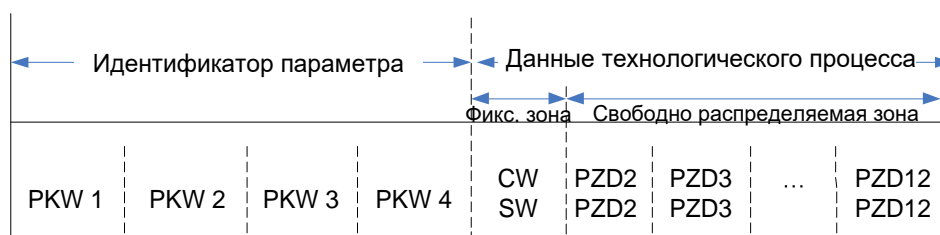
Рис. С.7 Структура сообщения PROFIBUS-DP
