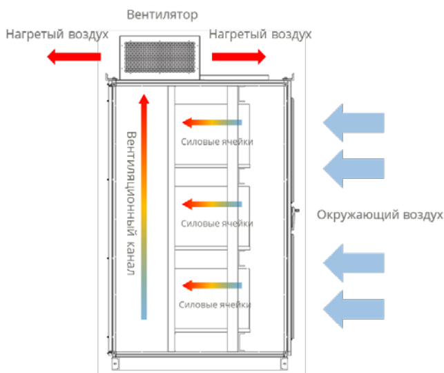
Рис. 8.9 Схема расположения воздухопроводов охлаждающего воздуха
