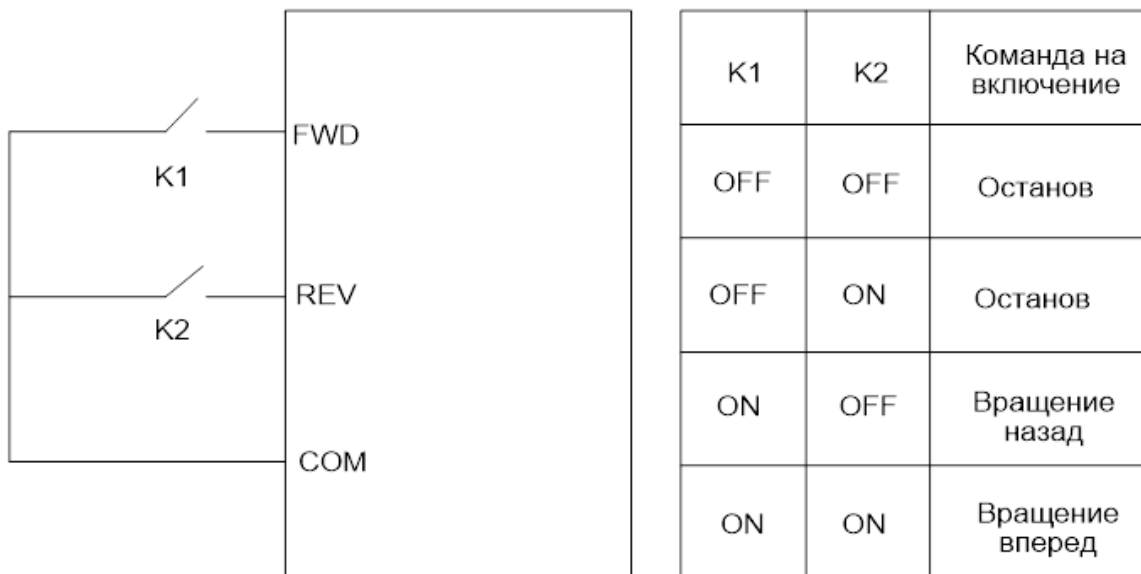
Рис. 5.16 Двухпроводное управление (раздельное управление включением и направлением вращения)
