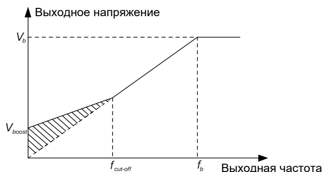
Рис. 6.3 Повышение момента
