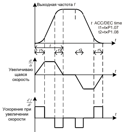
Рис. 5.4 Ускорение/торможение при S-образной характеристике
