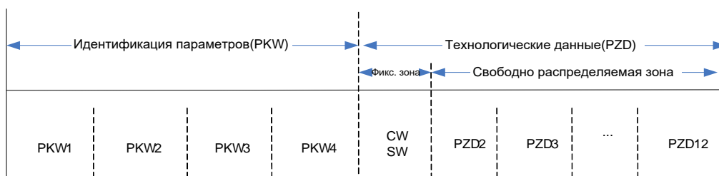
Рис. 5.36 Структура кадра данных в протоколе PROFIBUS-DP
