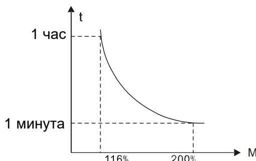
Рис. 5.33 Настройка коэффициента защиты двигателя от перегрузки
