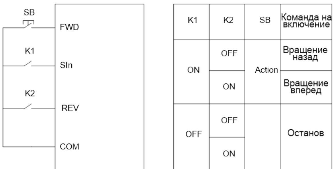
Рис. 5.17 Режим трехпроводного управления 1
