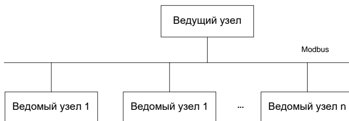
Рис. В.1 Топологическая структура коммуникационной сети MODBUS
