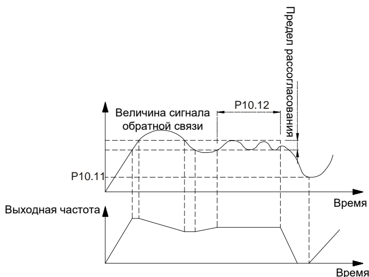
Рис. 5.27 Соотношение между предельным рассогласованием ПИД-регулятора и выходной частотой ПЧ
