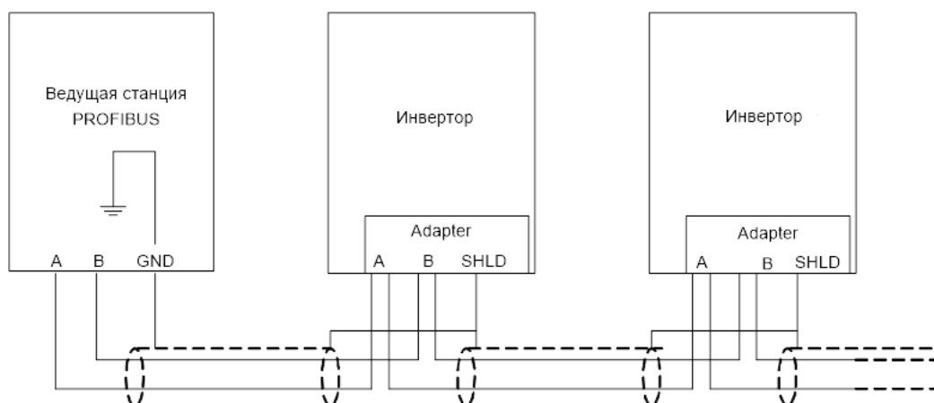
Рис. С.6 Стандартное подключение кабеля PROFIBUS
