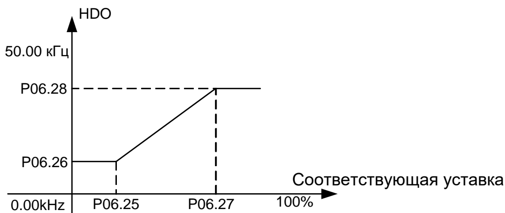
Рис. 5.20 Связь между HDO и соответствующей уставкой
