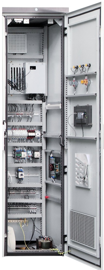
Рис. 3.8 Расположение компонентов в шкафу управления
