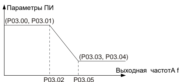
Рис. 5.8 Параметры пропорционально-интегрального управления
