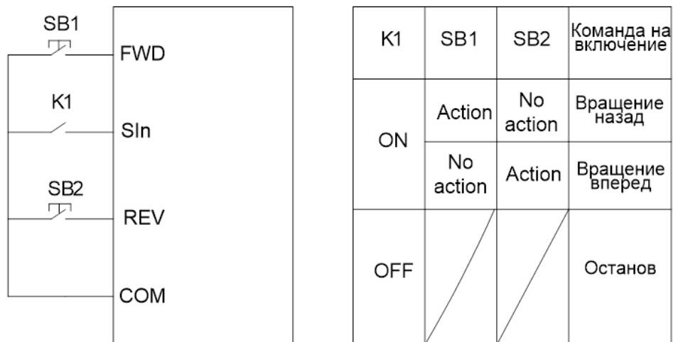
Рис. 5.18 Режим трехпроводного управления 2
