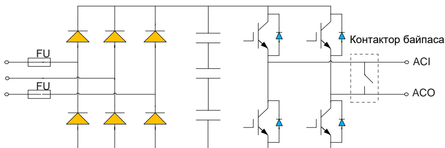
Рис. 3.2 Блок-схема силовых модулей
