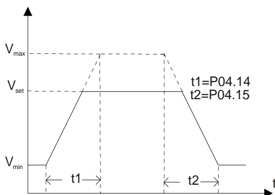
Рис. 5.12 Диаграмма настройки верхнего и нижнего предела напряжения
