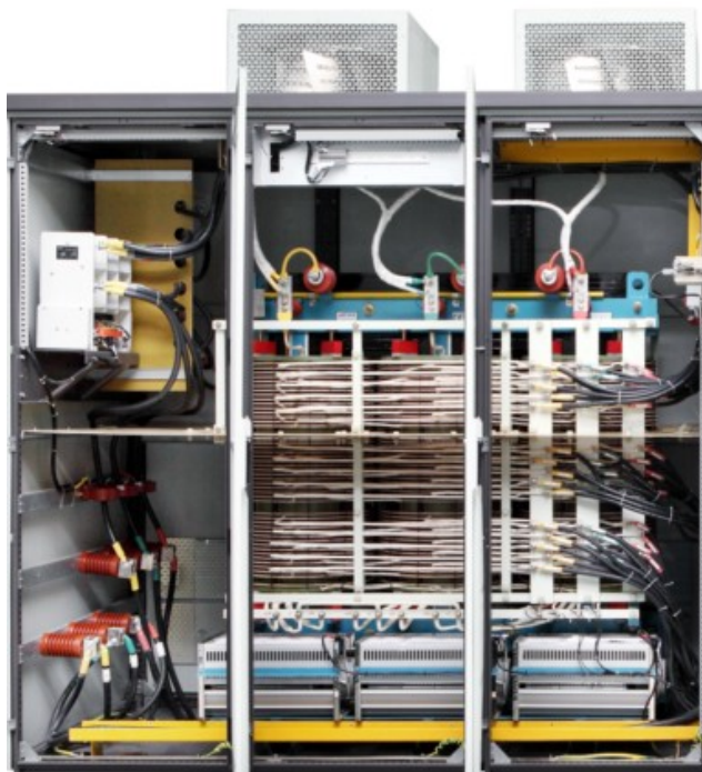
Рис. 3.6 Расположение компонентов в шкафу трансформатора
