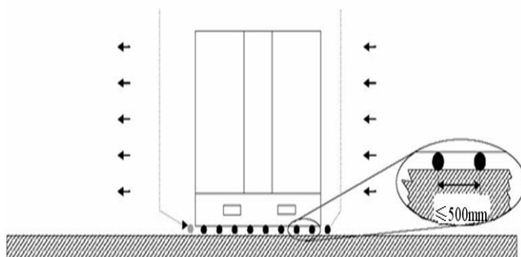
Рис. 8.4 Перемещение при помощи круглых подкладок
