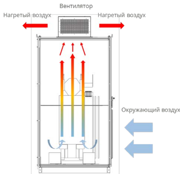
Рис. 8.8 схема испытания трансформаторного кабинета путь
