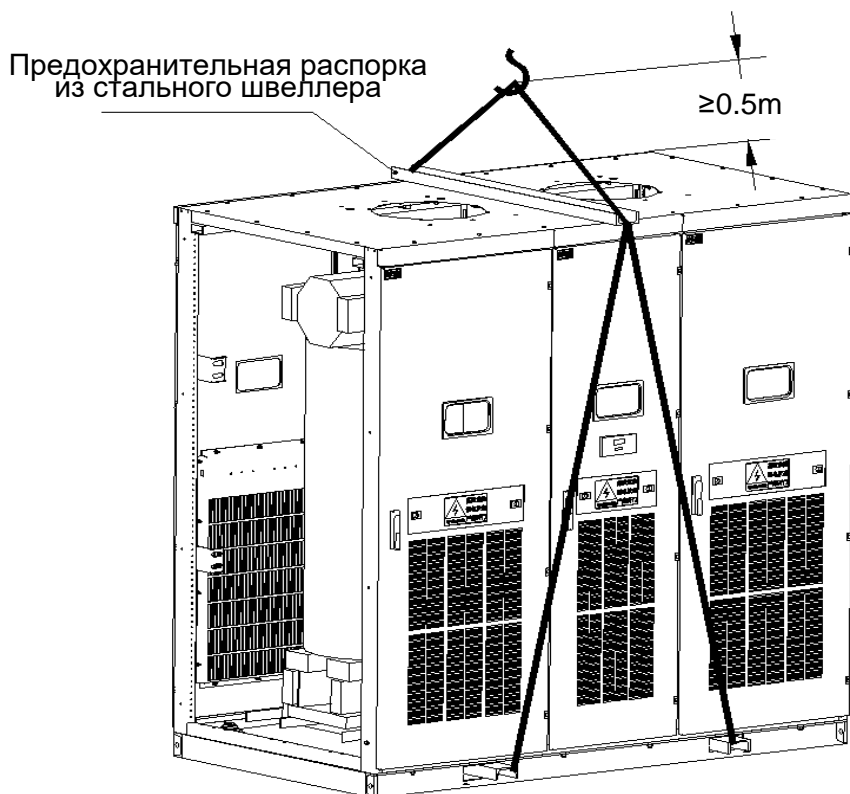
Рис. 8.2 Подъем шкафа в сборе
