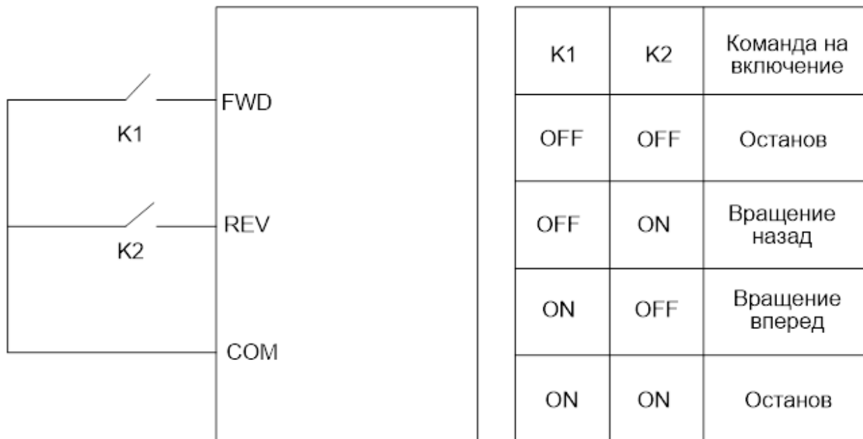
Рис. 5.15 Двухпроводное управление (объединенное управление включением и направлением вращения)
