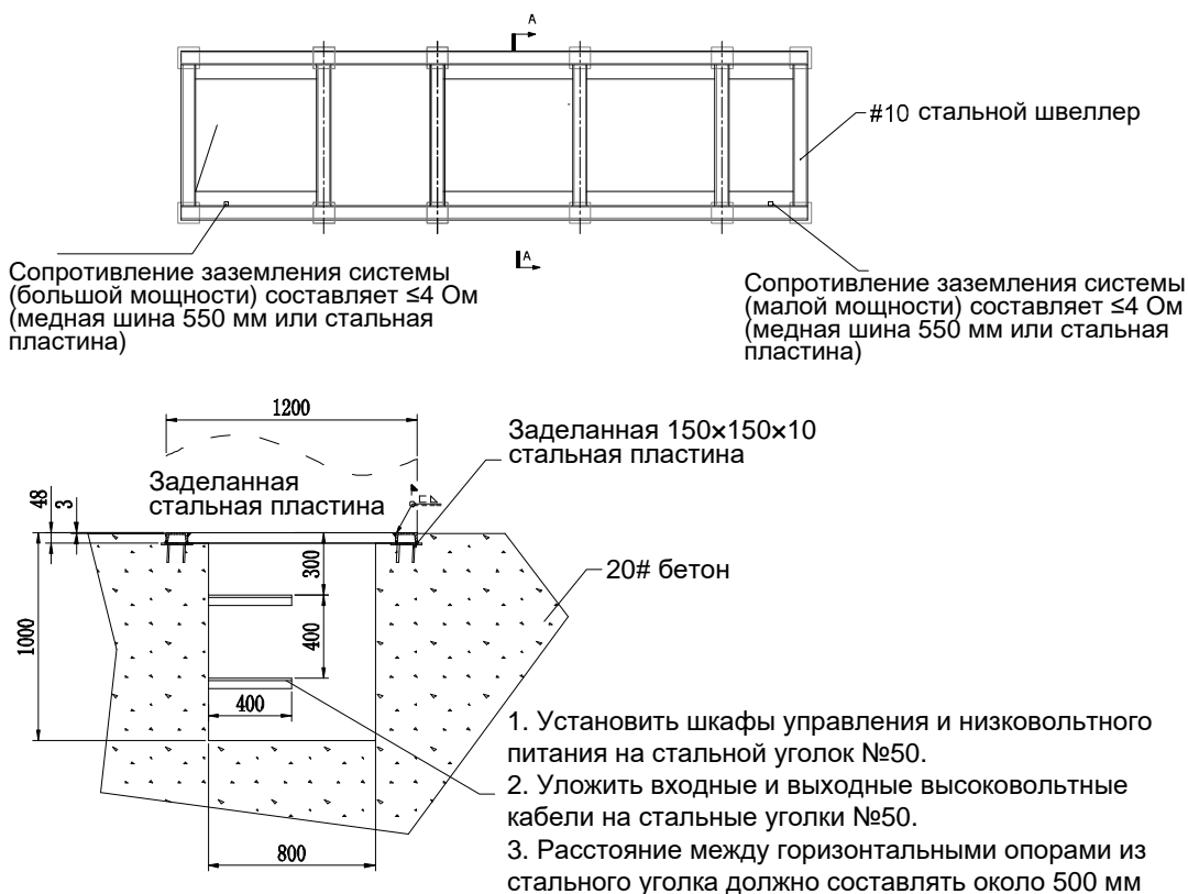
Рис. 8.10 Схема монтажного фундамента
