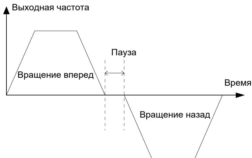
Рис. 5.6 Характеристика паузы при изменении направления вращения
