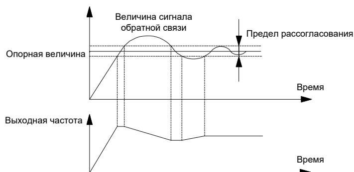
Рис. 5.28 Схема режима бездействия и выхода из него
