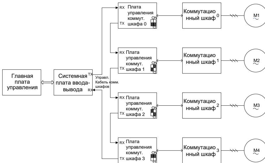
Рис. 3.4 Компоновка коммутационных шкафов
