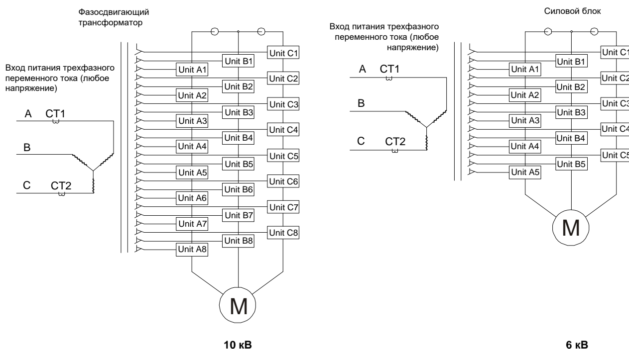
Рис. 3.1 Топологическая схема
