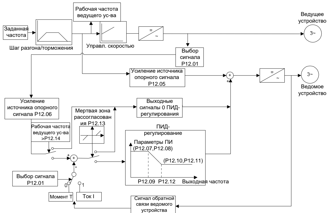
Рис. 5.30 Схема гибкого подключения «ведущее-ведомое устройство», ведомое устройство находится в режиме управления скоростью вращения
