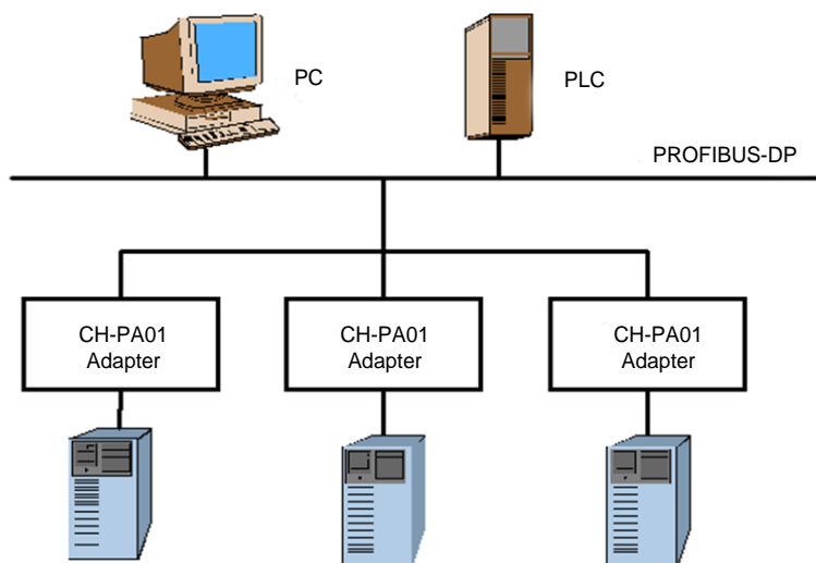
Рис. С.1 Топология шины PROFIBUS
