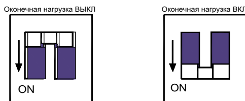
Рис. С.5 Оконечная нагрузка шины
