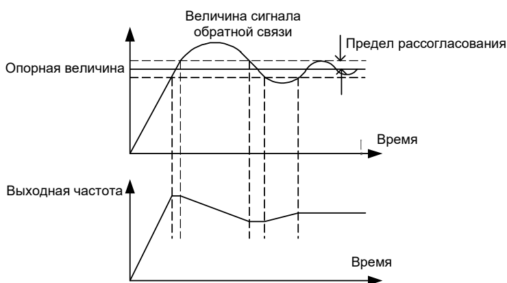
Рис. 5.32 Предел рассогласования и соответствующая выходная частота
