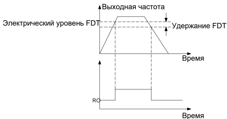
Рис. 5.23 Диаграмма электрического уровня FDT
