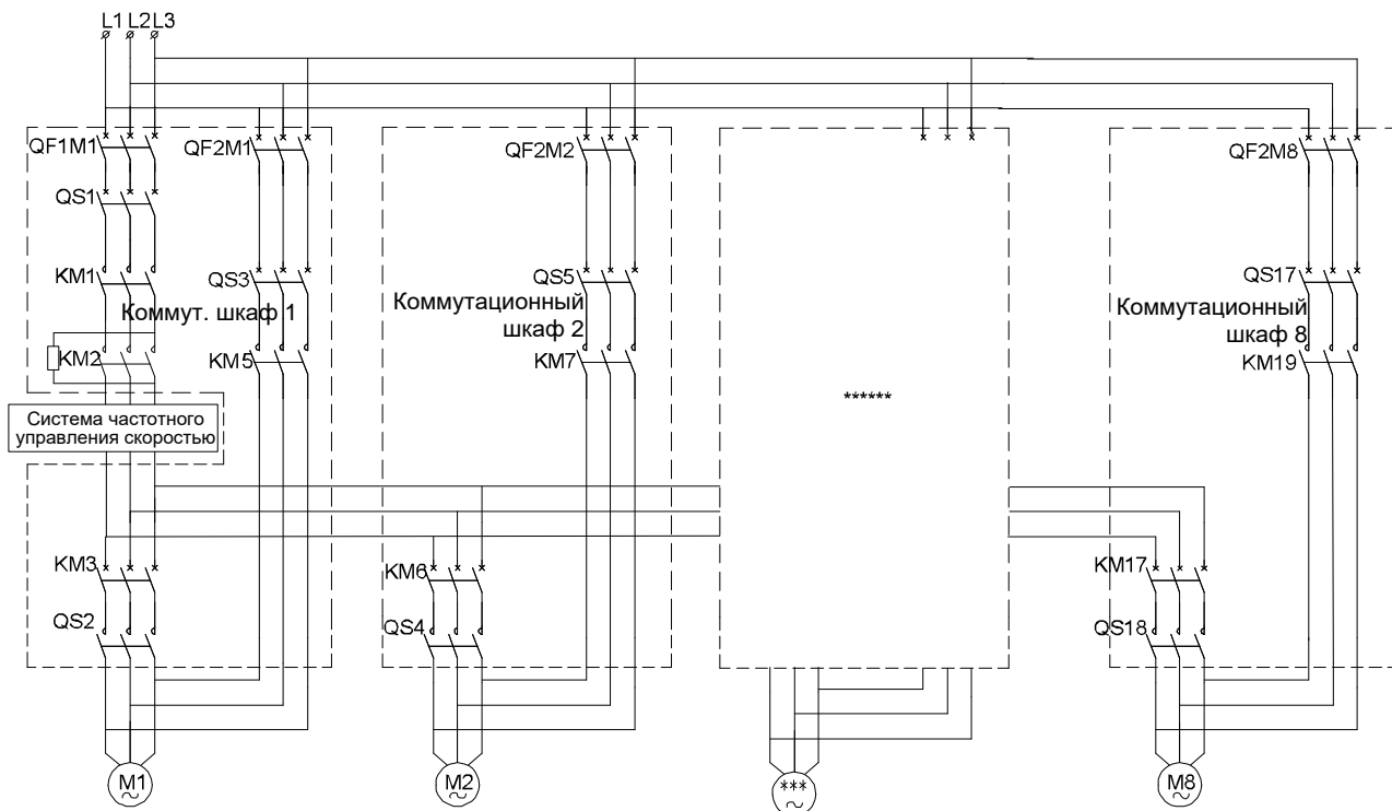
Рис. 5.14 Схема системы управления несколькими приводами
