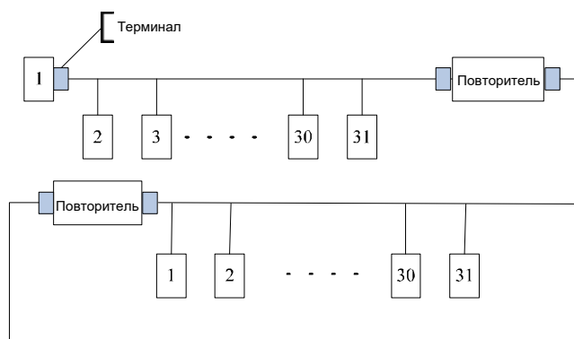
Рис. С.4 До 32 станций в каждом сегменте
