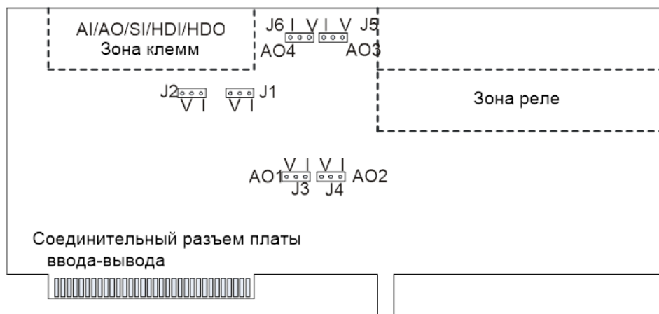
Рис. 3.3 Коммутационные перемычки на плате ввода-вывода
