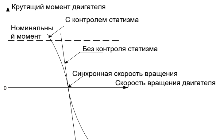
Рис. 5.25 Схема контроля статизма
