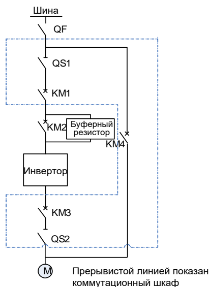
Рис. 5.13 Схема коммутации
