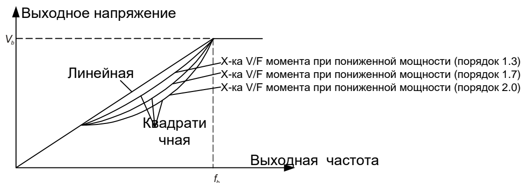
Рис. 5.9 Характеристики V/F
