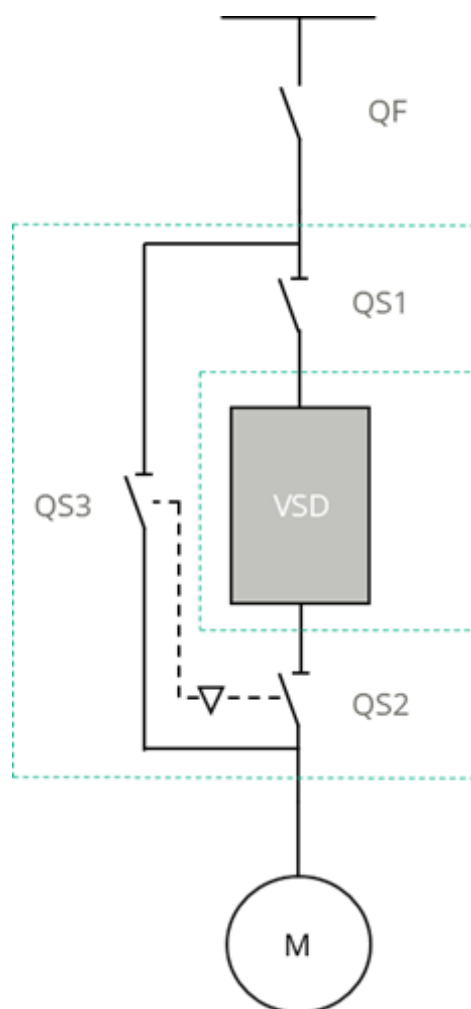
Рис. 3.9 Схема основных цепей шкафа ручного байпаса
