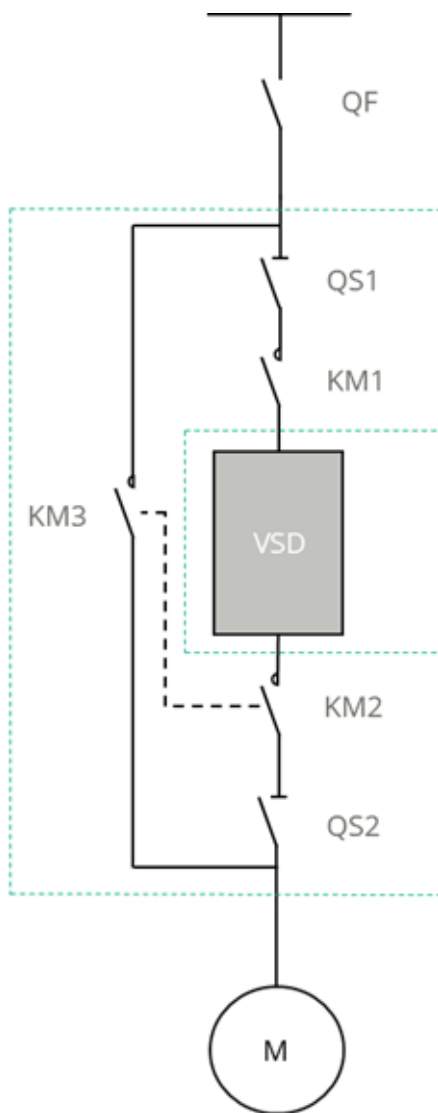
Рис. 3.10 Схема основных цепей шкафа автоматического байпаса
