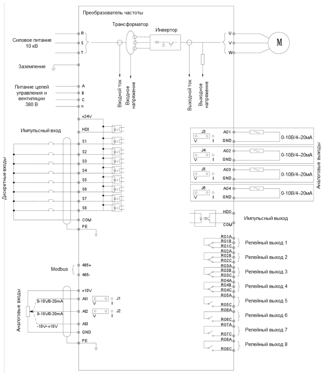
Рис. 4.2 Схема подключения цепей управления
