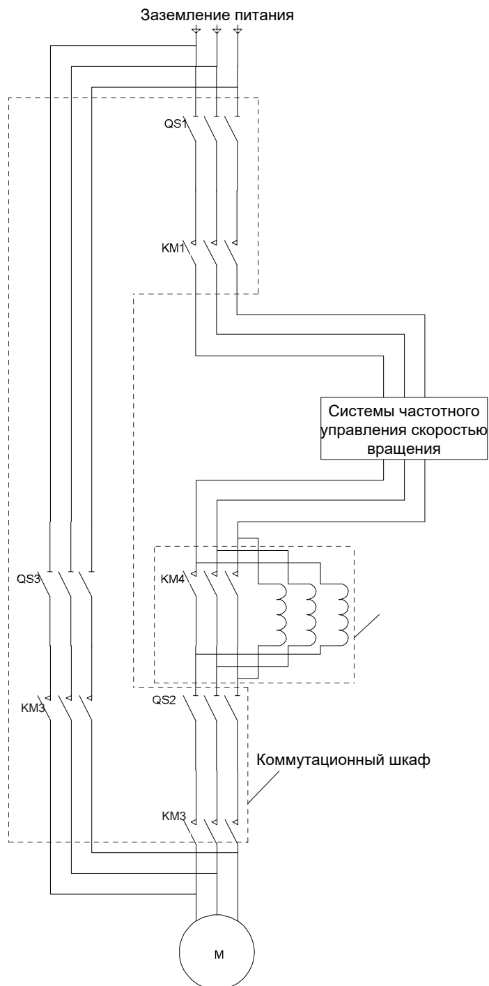
Рис. 6.4 Схема синхронного переключения
