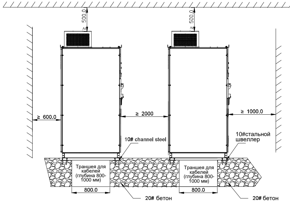
Рис. 8.7 Монтажная схема 3 при двухрядном расположении (вид сбоку, ед. измерения: мм)
