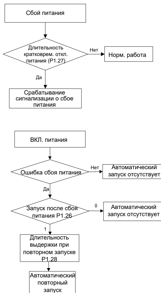
Рис. 5.7 Повторный запуск после отключения питания
