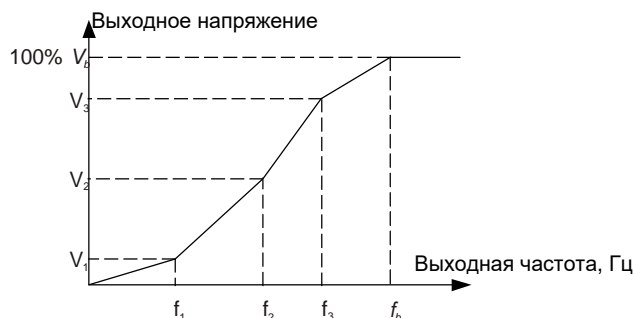
Рис. 5.11 Диаграмма настройки характеристики V/F
