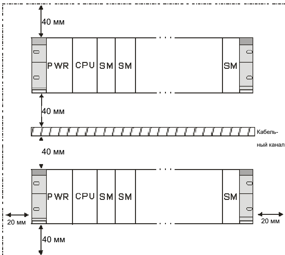
Рисунок 1-4. Схема установки
