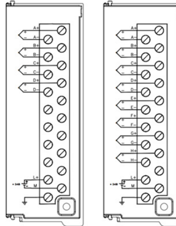
Расположение клемм входных каналов: слева SM3T14TC, справа SM3T18TC
