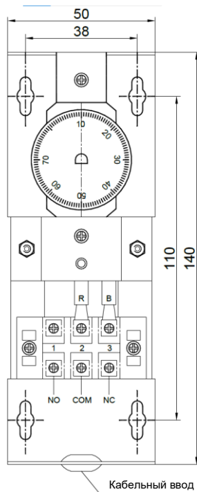
Габаритные и установочные размеры, мм
