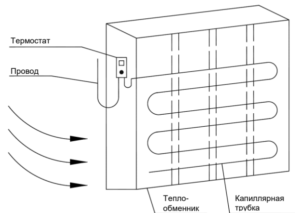
Схема установки
