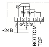
VGFA018F VGFA030F
