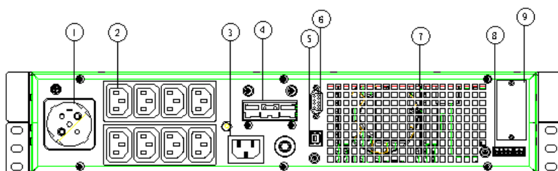
Рисунок 7-2. Задняя панель (1кВА)
