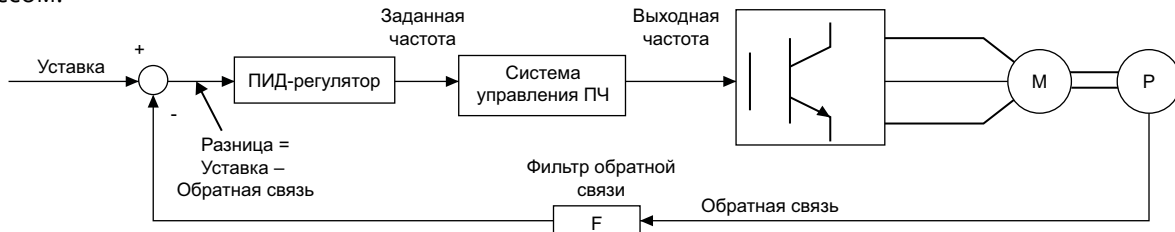
Рисунок 4-24 Блок-схема ПИД-регулирования
