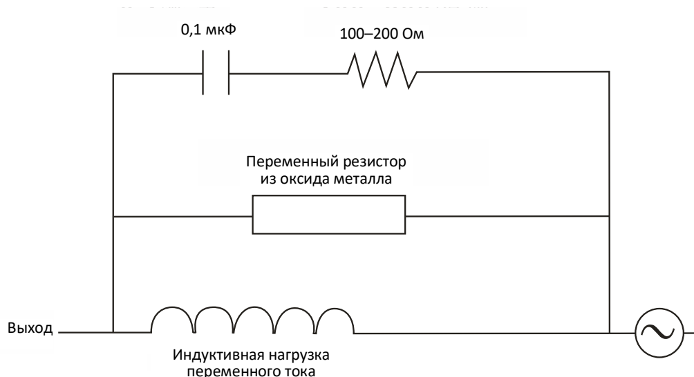
Рисунок 1-6. Цепь подавления нагрузки переменного тока
