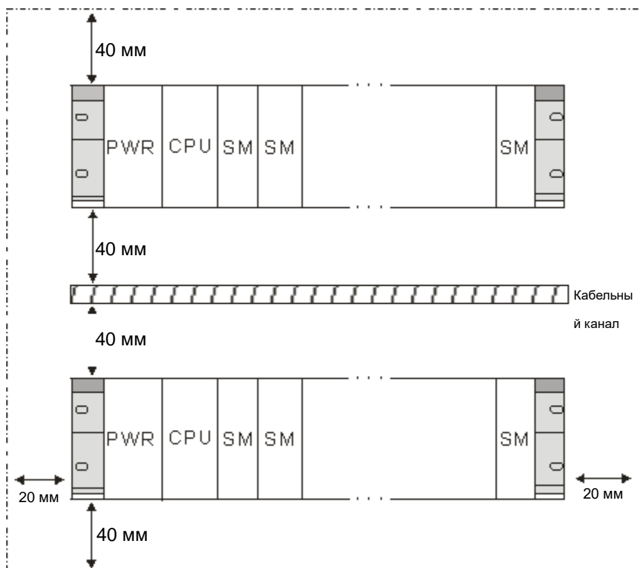
Рисунок 1-4. Схема установки
