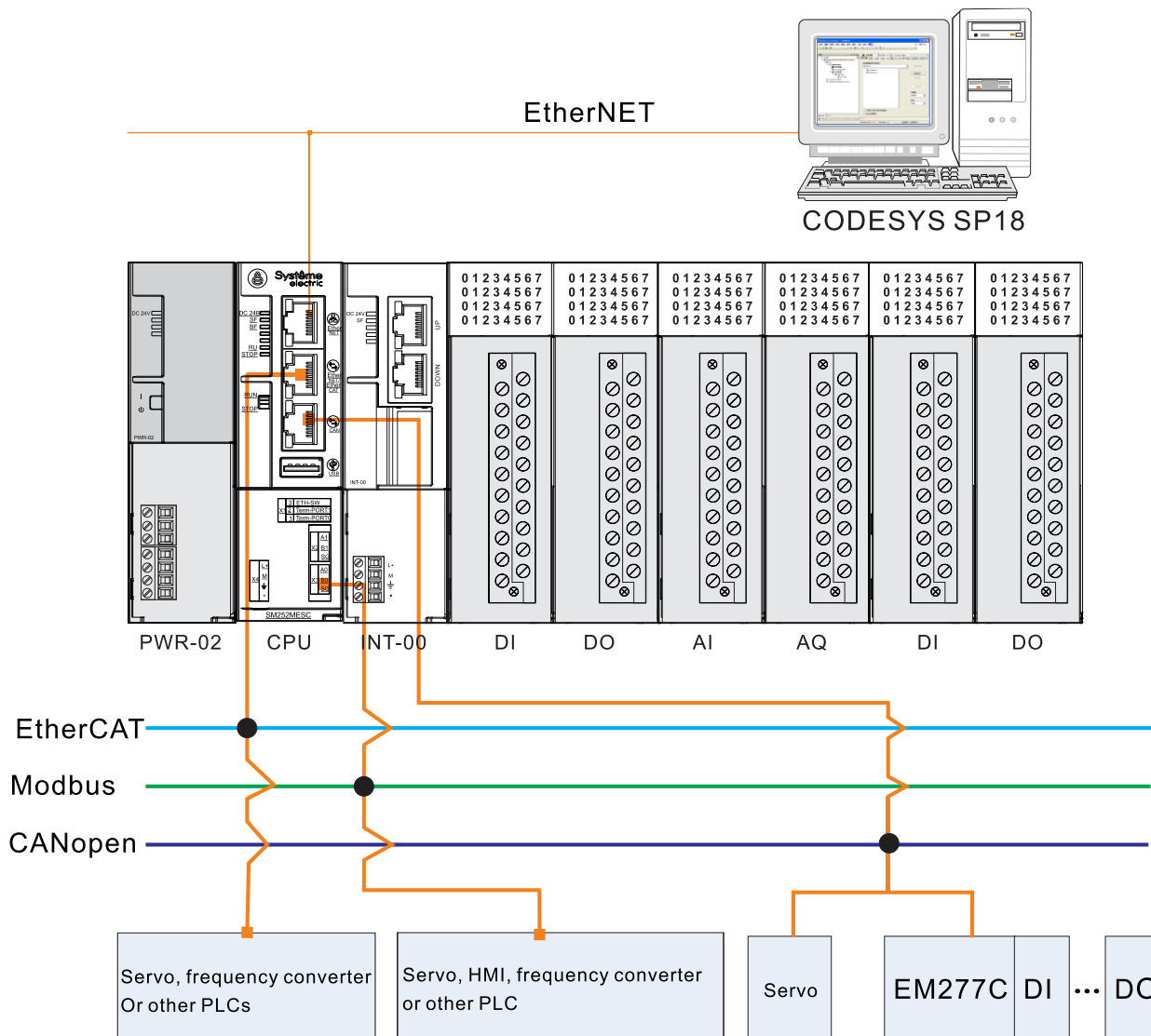
Рисунок 1-3. Схема сетевой архитектуры SM252MESC
