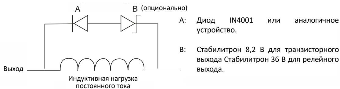
Рисунок 1-5. Цепь подавления нагрузки постоянного тока
