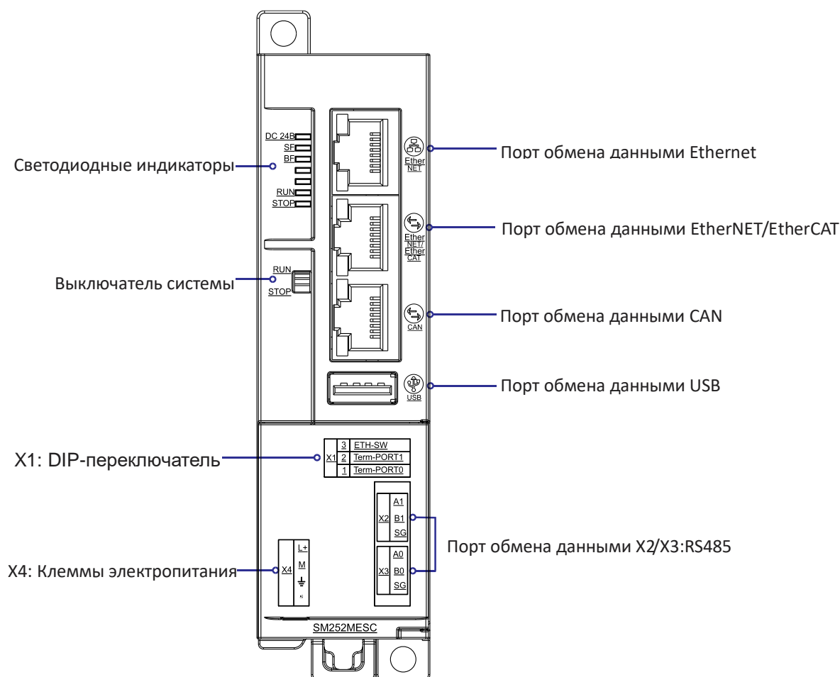
Рисунок 1-1. Схема внешнего вида интерфейсов SM252MESC
