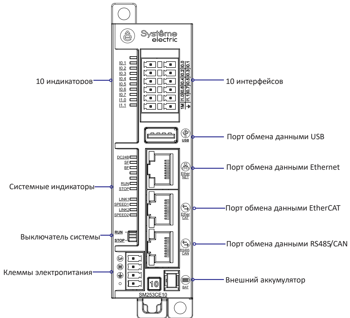
Рисунок 1-2. Схема внешних интерфейсов SM253CE10
