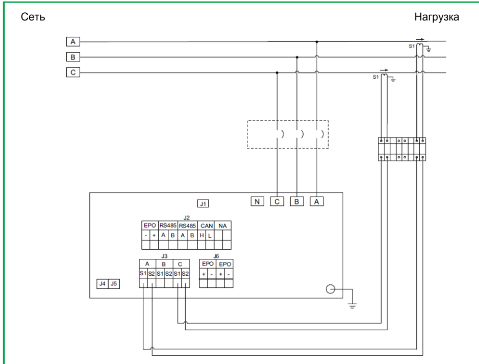
Рис. 6.3.3.5 Схема подключения ТТ со стороны нагрузки (без нейтрали)
