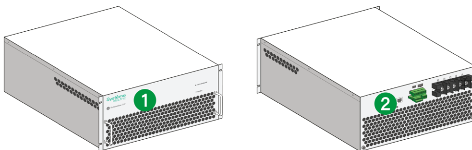
1 – Светодиодная индикация состояния модуля 2 – Интерфейс для подключения модуля
