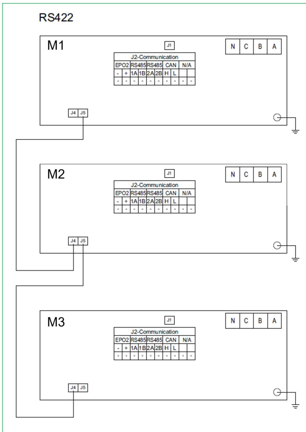
Рис. 6.4.2.5 Подключение RS422 при параллельном режиме работы
