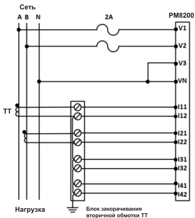
1-фазное 3-проводное прямое подключение по схеме «расщеплённая фаза» (2 трансформатора тока)
