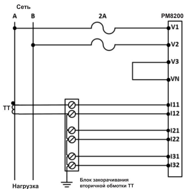
1-фазное 2-проводное прямое L-L подключение (1 трансформатор тока)
