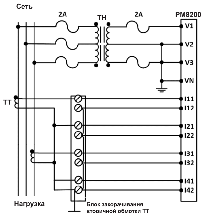
3-фазное 3-проводное трансформаторное подключение по схеме «разомкнутый треугольник» (2 трансформатора напряжения и 2 трансформатора тока)
