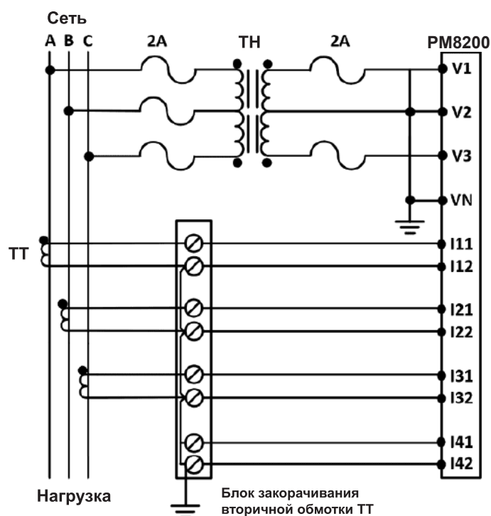
3-фазное 3-проводное трансформаторное подключение по схеме «разомкнутый треугольник» (2 трансформатора напряжения и 3 трансформатора тока)
