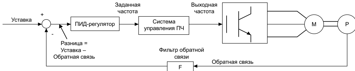
Рисунок 4-24 Блок-схема ПИД-регулирования
